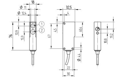
Kabelversion / Version with cable / Version avec câble
