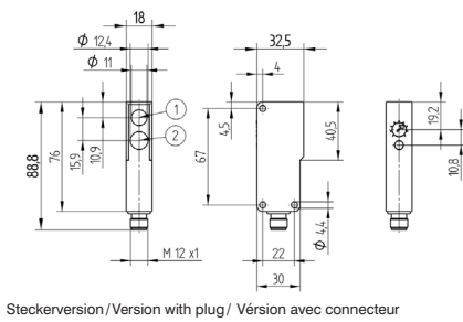
Steckversion / Version with plug / Version avec connecteur
