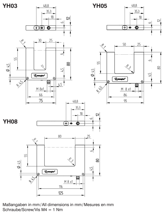
Gabellichtschranke Fork Sensor Fourche optique
