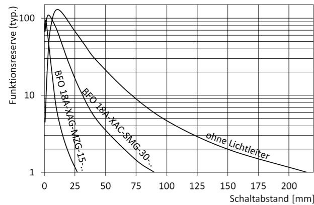
Bild 7: Funktionsreserve in Abhängigkeit vom Abstand für BFB M18M-012-P-S4, Bezugsmaterial weiß, 90 % Remission, 100 x 100 mm 2
