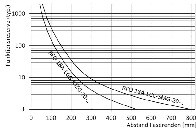
Bild 8: Funktionsreserve in Abhängigkeit vom Abstand der Faserköpfe für BFB M18M-011-P-S4
