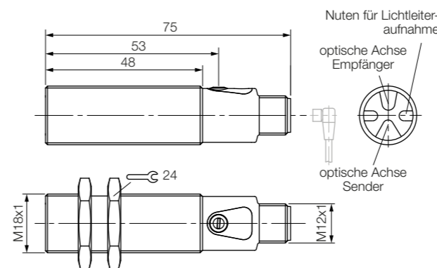
Bild 2: Abmessungen
