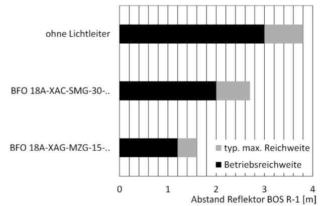
Bild 12: Funktionsdiagramm für BFB M18M-011-P-S4, Bezugsmaterial Reflektor BOS R-1
