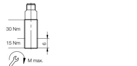
Bild 3: Zulässige Anzugsdrehmomente
