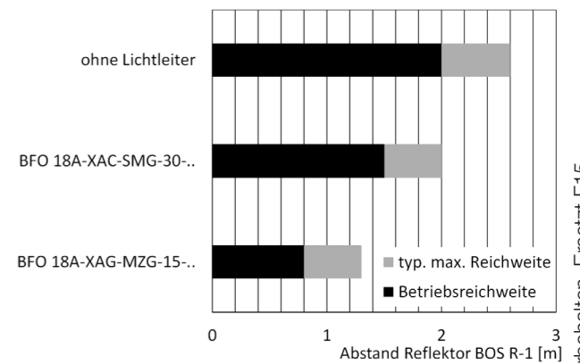
Bild 13: Funktionsdiagramm für BFB M18M-012-P-S4, Bezugsmaterial Reflektor BOS R-1
