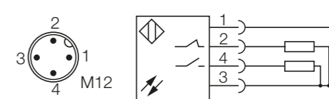
Bild 5: Steckerbild, Anschluss-Schaltbild
