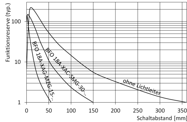
Bild 6: Funktionsreserve in Abhängigkeit vom Abstand für BFB M18M-011-P-S4, Bezugsmaterial weiß, 90 % Remission, 100 x 100 mm 2
