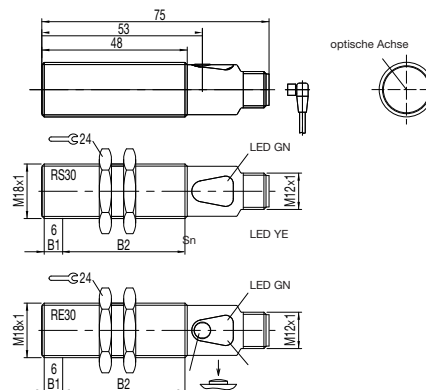
Bild 4: Abmessungen, Anzugsdrehmoment B1 = 15 Nm, B2 = 30 Nm
