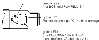
Bild 3: Anzeige- und Bedienelemente
