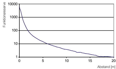
Bild 7: Funktionsreserve in Abhängigkeit vom Abstand. Bezugsmaterial weiß, 90 % Reflexion, 200 x 200 mm 2
