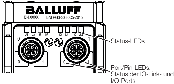
Bild 4-3: Anzeigeelemente
