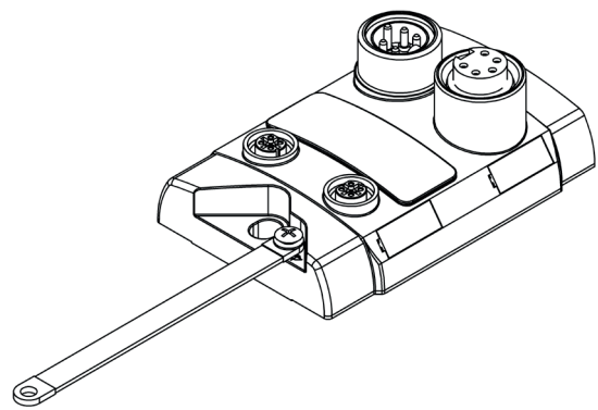
Bild 5-4: Anschluss Erdung
