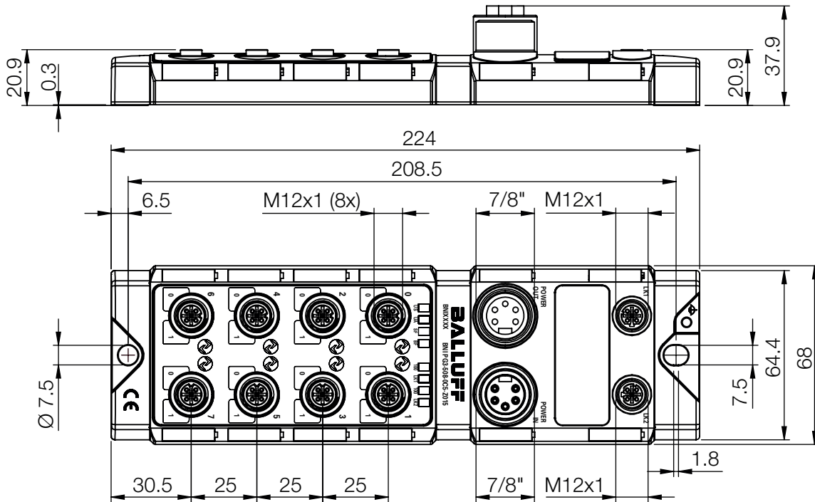
Bild 4-1: Abmessungen, Aufbau und Funktion
