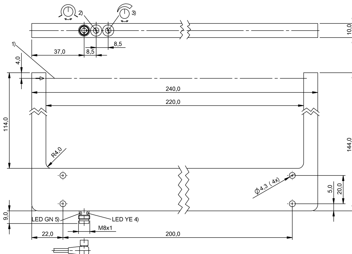
1) Oś optyczna 2) Czułość 3) Przełączanie "na jasno"/"na ciemno" 4) Funkcja wyjścia 5) Napięcie robocze
