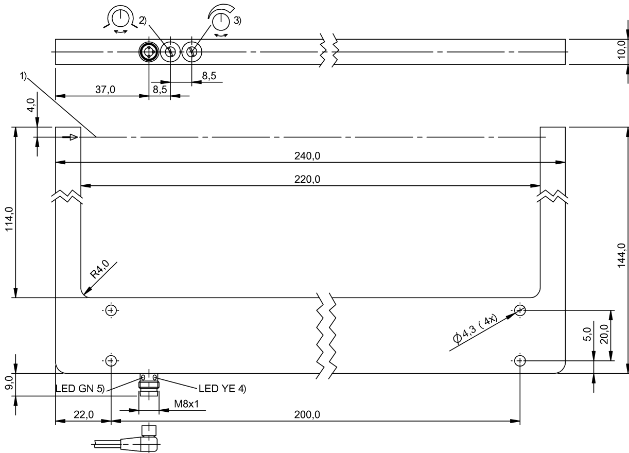
1) Oś optyczna 2) Czulość 3) Przelączenie "na jasno"/"na ciemno" 4) Funkcja wyjścia 5) Napięcie robocze
