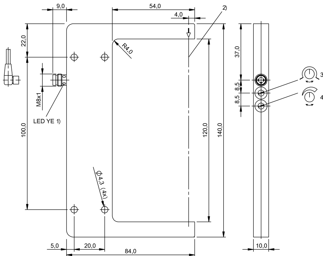
1) Funkcja wyjścia 2) Oś optyczna 3) Przełączanie "na jasno"/"na ciemno" 4) Czulość
