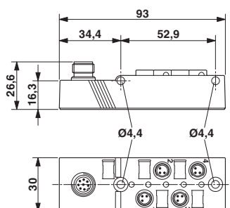
Rysunek wymiarowy
