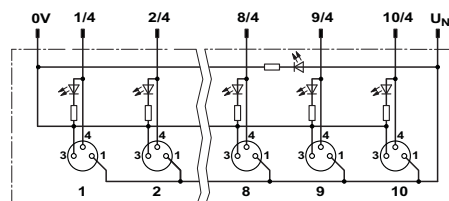
Schemat
