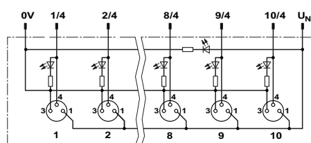
Schemat
