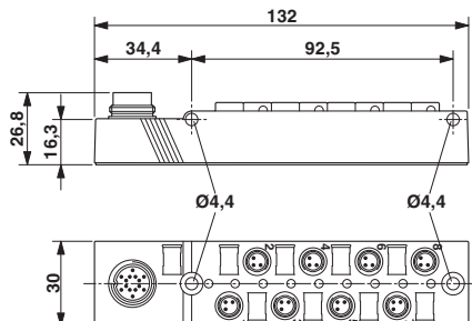
Rysunek wymiarowy
