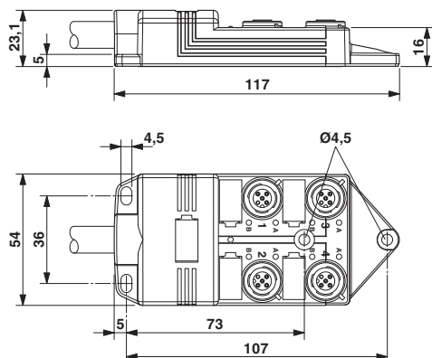
Rysunek wymiarowy
