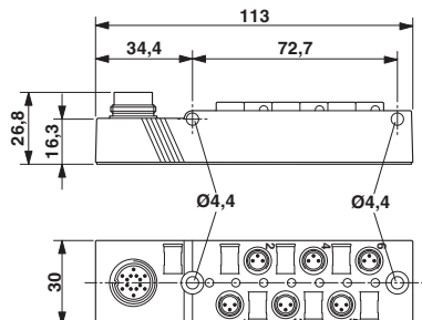
Rysunek wymiarowy
