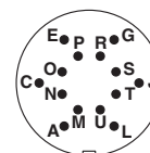
Przyłącze wtykowe M16, wtyk 14-biegunowy
