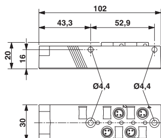
Rysunek wymiarowy
