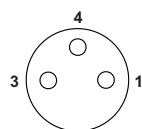
Gniazdo rozszerzeń M8, 3-biegunowe
