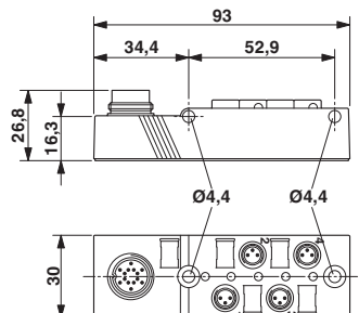
Rysunek wymiarowy
