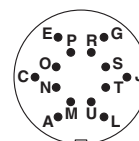
Układ styków M16, przyłącze wtykowe 14-biegunowe
