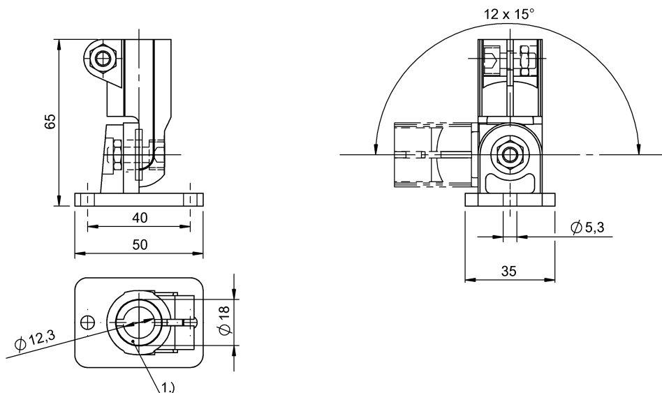
1) Tuleja redukcyjna
