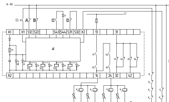
Rys. 3: SRB202CA, 202CA/T, SRB202CA/Q, SRB202CA/QT
