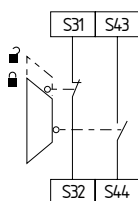
Rys. 13 SRB202CA, SRB202CA/T, SRB202CA/Q, SRB202CA/QT
