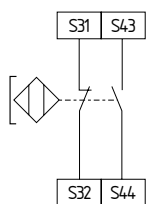
Rys. 14 SRB202CA, SRB202CA/T, SRB202CA/Q, SRB202CA/QT
