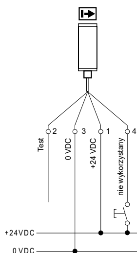
Konfiguracja przyłączy Nadajnik
