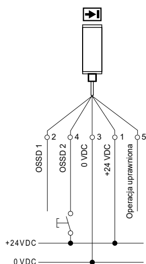
Konfiguracja przyłączy Odbiornik
