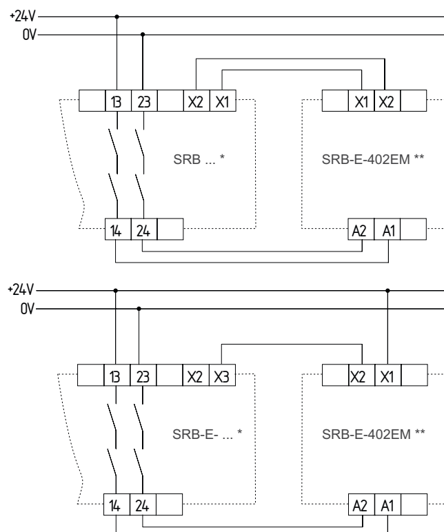
Rys. 4 * = Moduł podstawowy; ** = Moduł rozszerzeń
