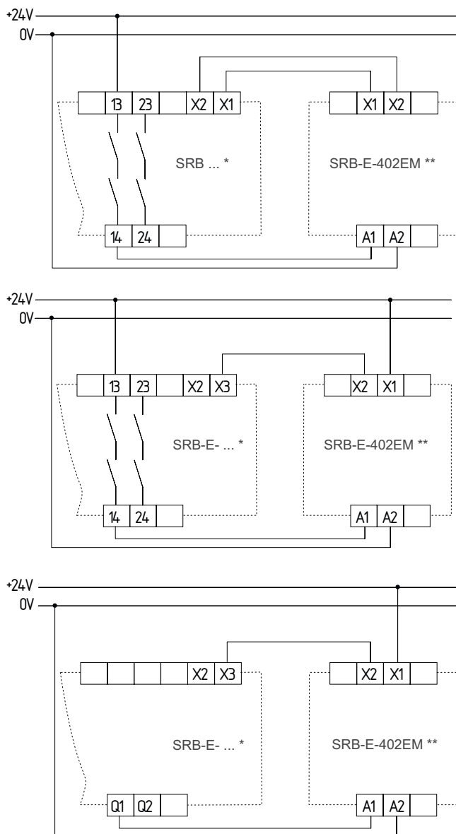
Rys. 3 * = Moduł podstawowy; ** = Moduł rozszerzeń
