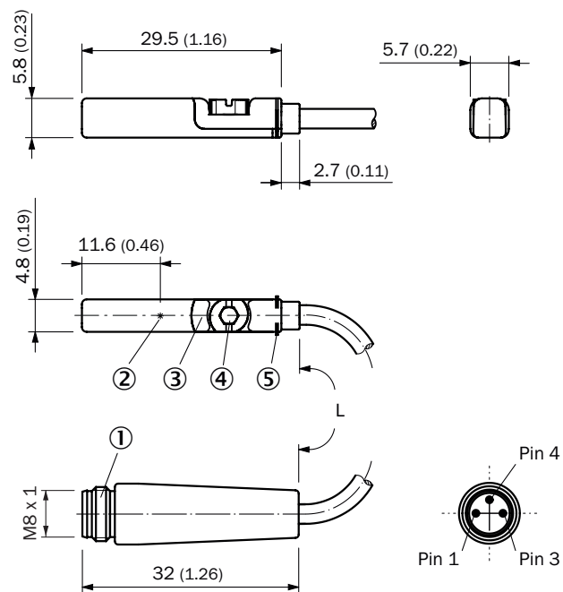
Rysunek wymiarowy Przewód z wtykiem M8
