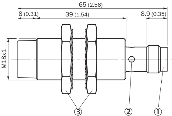
Rysunek wymiarowy IMB18 Standard, wtyk M12, niezabudowany
