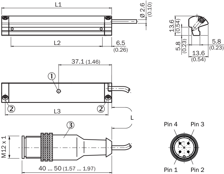
Rysunek wymiarowy Przewód z wtykiem M12, ze złączem radełkowym
