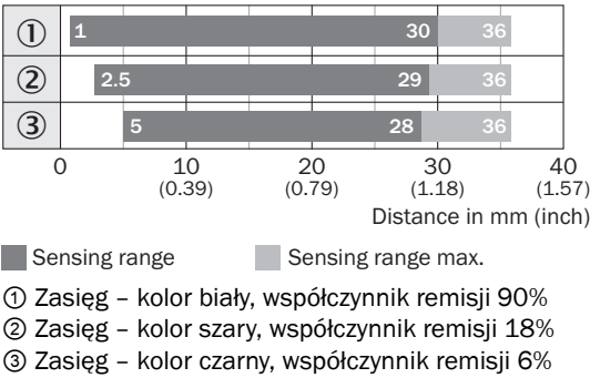
Wykres zasięgu wykrywania GTB2S, 30 mm
