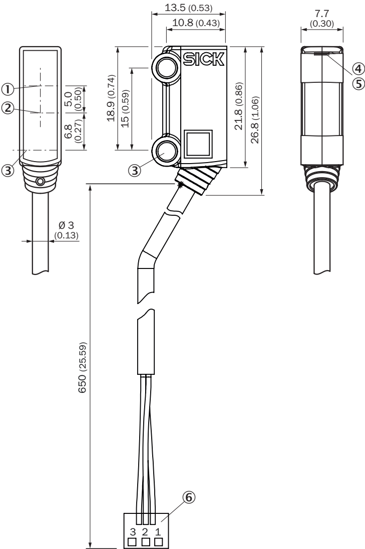
Rysunek wymiarowy
