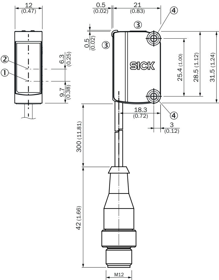
Rysunek wymiarowy
