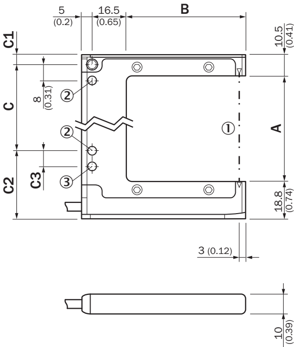
Rysunek wymiarowy WFE-xxxxxx1xx
