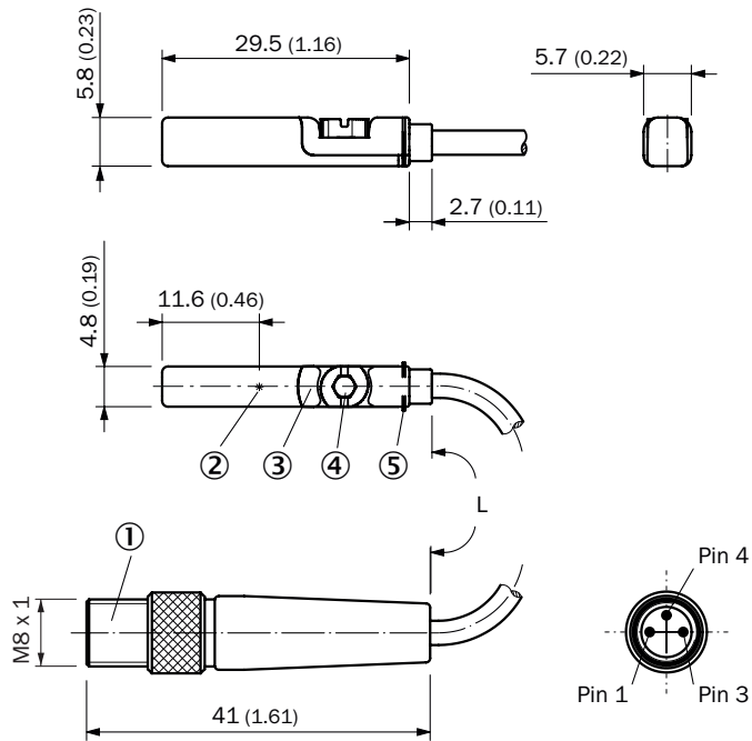
Rysunek wymiarowy Przewód z wtykiem, M8, ze złączem radełkowanym
