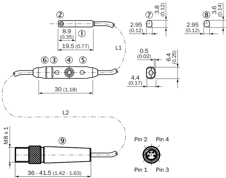
Rysunek wymiarowy Przewód z wtykiem, M8, ze złączem radełkowym
