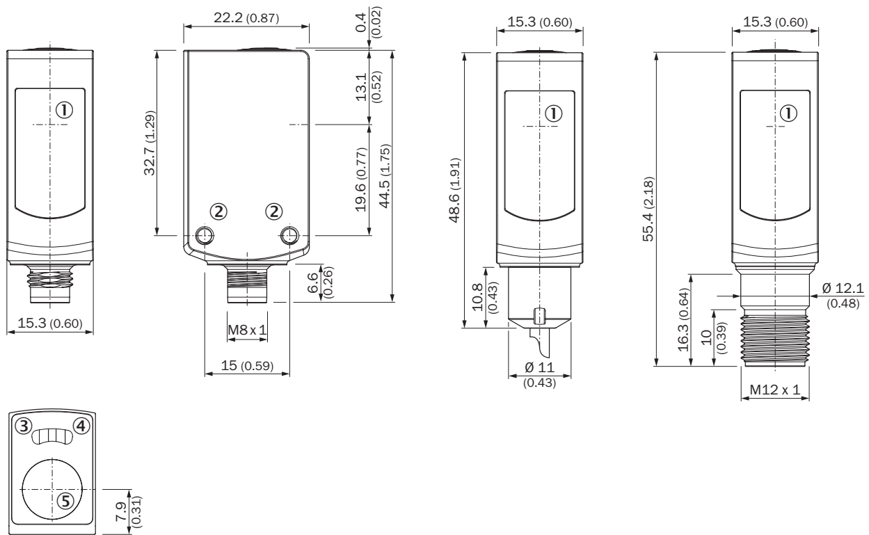
Rysunek wymiarowy WLG4S-3V, WLG4S-3V, z przyciskiem Teach-in
