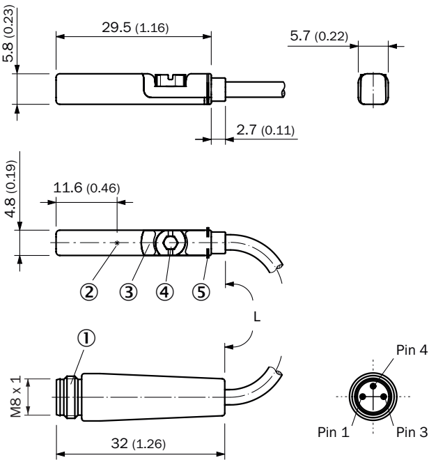
Rysunek wymiarowy Przewód z wtykiem M8
