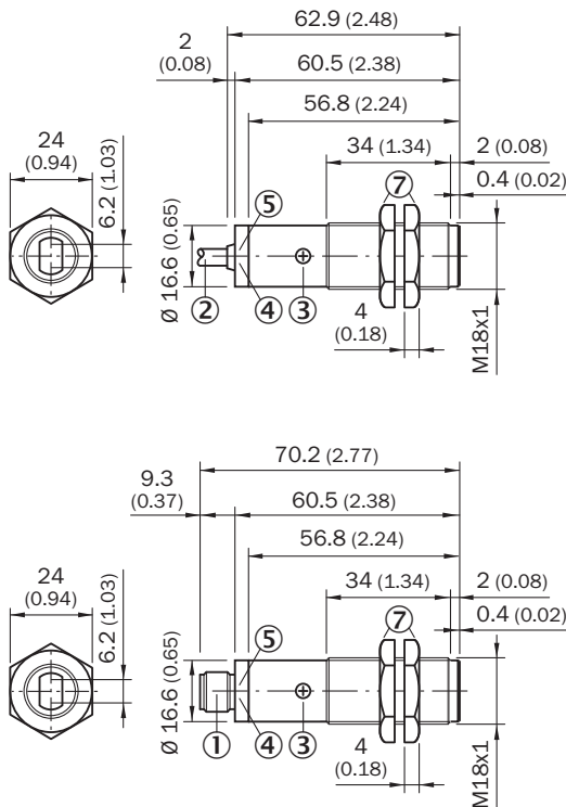
Rysunek wymiarowy VL180-2, metal, osiowy
