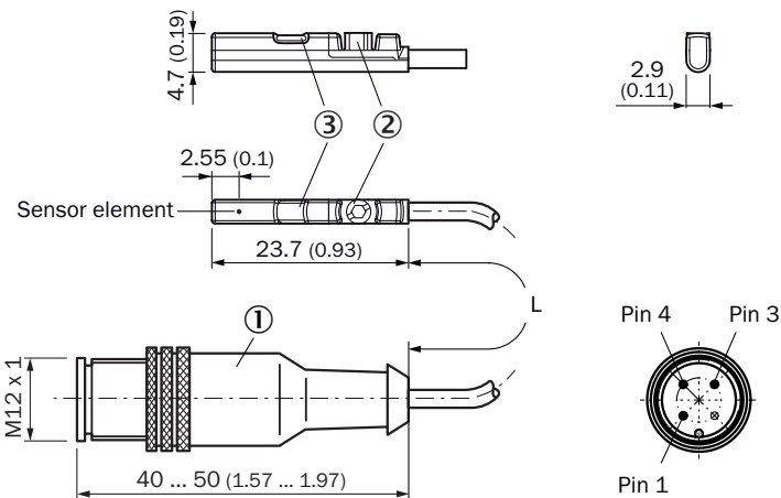
Rysunek wymiarowy Przewód z wtykiem M12
