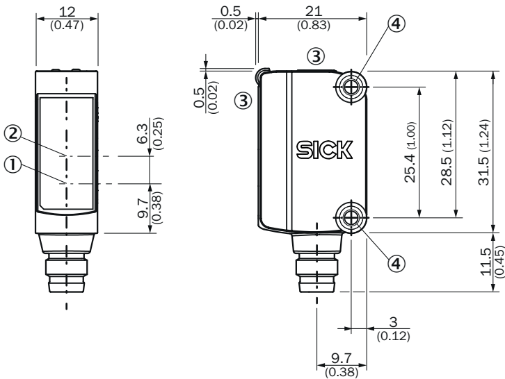
Rysunek wymiarowy
