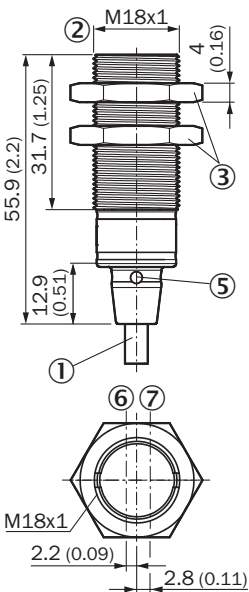
Rysunek wymiarowy GR18S Inox, przewód, osiowy
