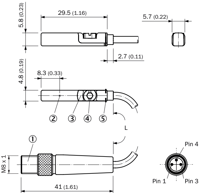
Rysunek wymiarowy Przewód z wtykiem, M8, ze złączem radełkowym
