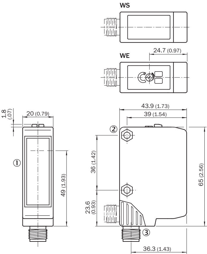
Rysunek wymiarowy WSE250-2, DC, wtyk
