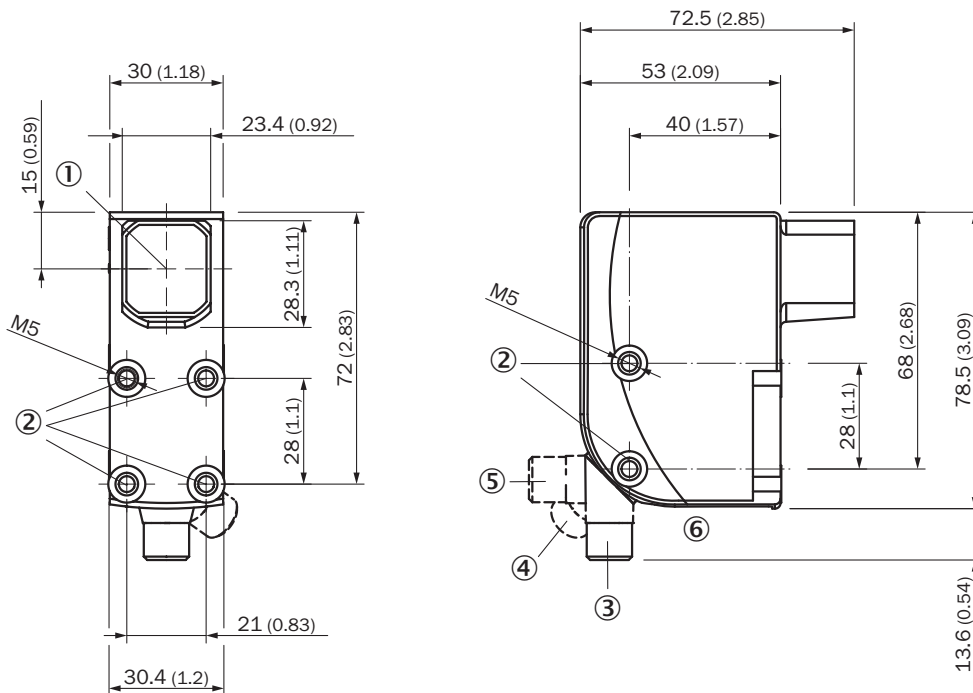
Rysunek wymiarowy Sensing distance from leading edge of lens
