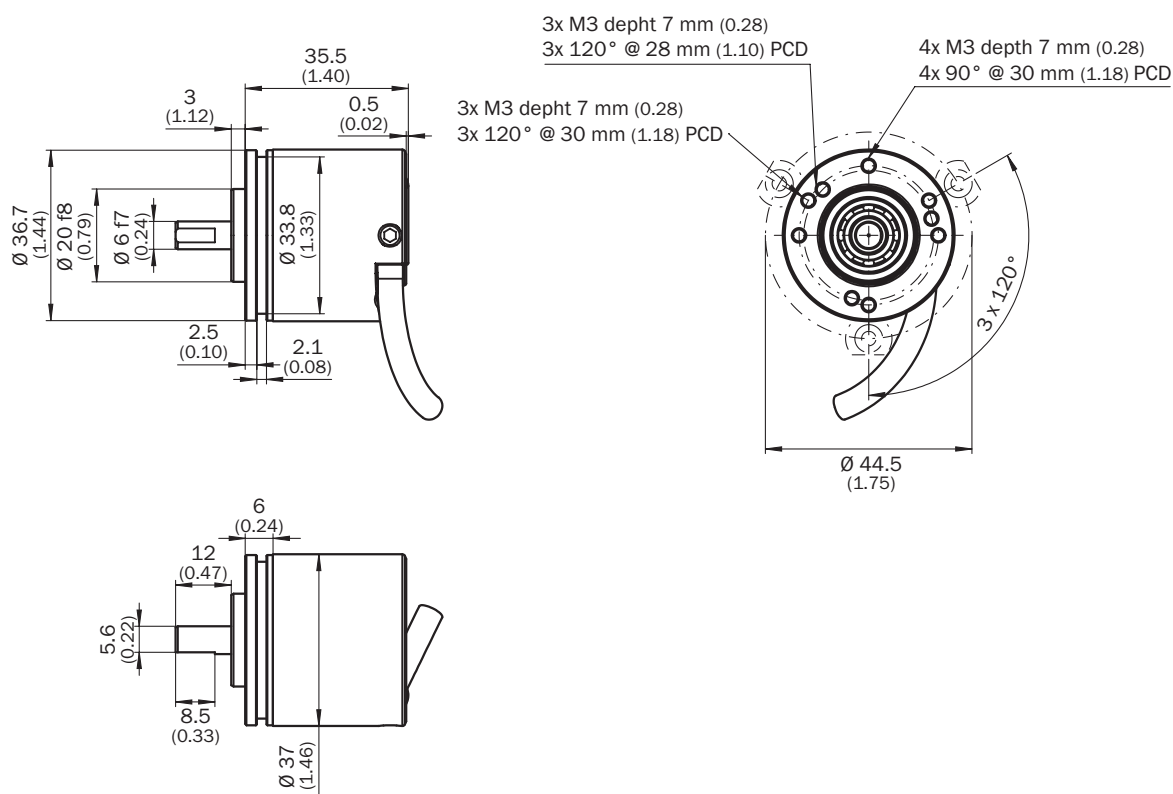
Rysunek wymiarowy Wałek, kołnierz zaciskowy, wałek 6 mm x 12 mm, układ otworów – wersja kołnierza – typ 0
