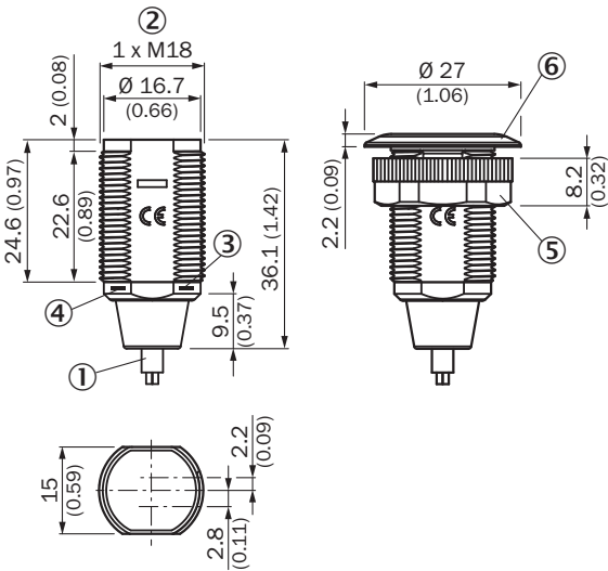
Rysunek wymiarowy GR18S, tworzywo sztuczne, przewód z wtykiem, osiowy
