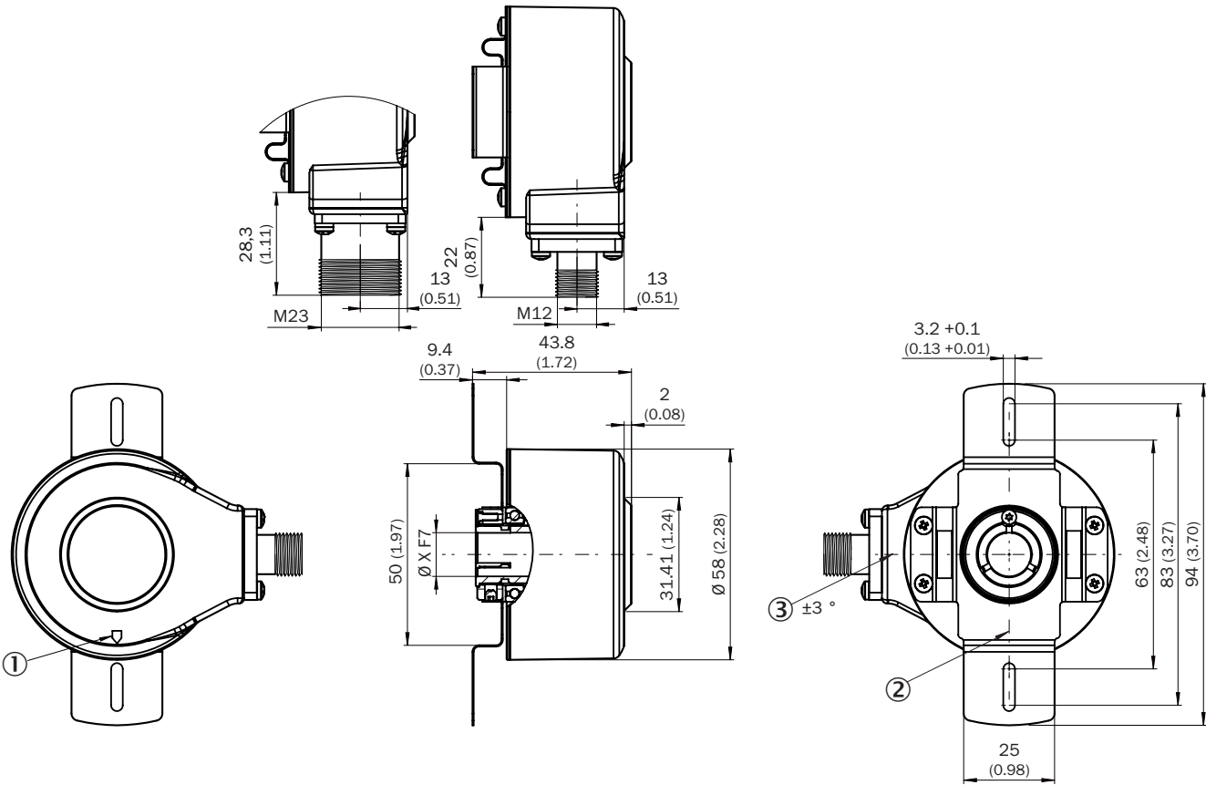
Rysunek wymiarowy
