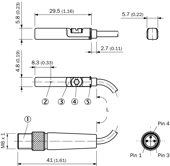
Rysunek wymiarowy Przewód z wtykiem, M8, ze złączem radełkowym
