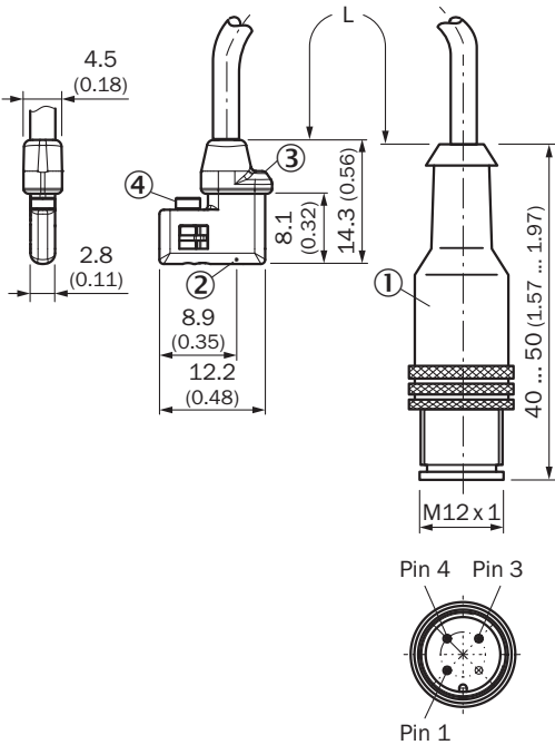
Rysunek wymiarowy Przewód z wtykiem M12, ze złączem radełkowym
