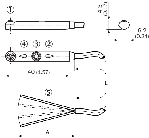
Rysunek wymiarowy Przewód
