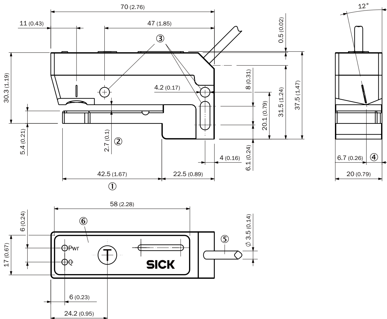
Rysunek wymiarowy, czujnik
