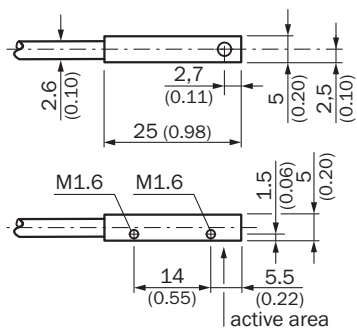
Rysunek wymiarowy IQ05
