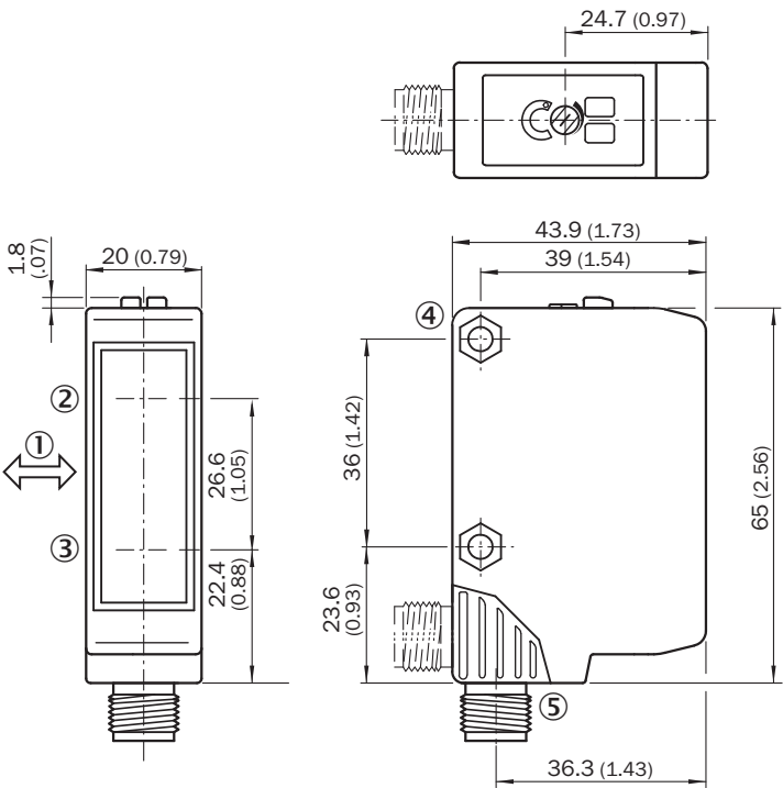
Rysunek wymiarowy WTB250-2, DC, wtyk
