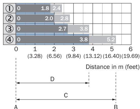
Wykres zasięgu wykrywania Precyzyjne odbłyśniki trzypolowe
