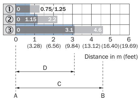
Wykres zasięgu wykrywania Folia odbłaskowa
