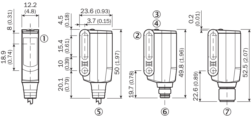
Rysunek wymiarowy WL9M4-3, WSE9M4-3
