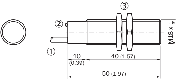
Rysunek wymiarowy MM18, przewód, standardowy
