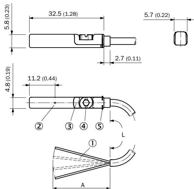
Rysunek wymiarowy Przewód
